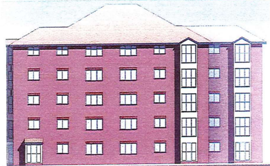
3 Elevation 3 - a 1:100
