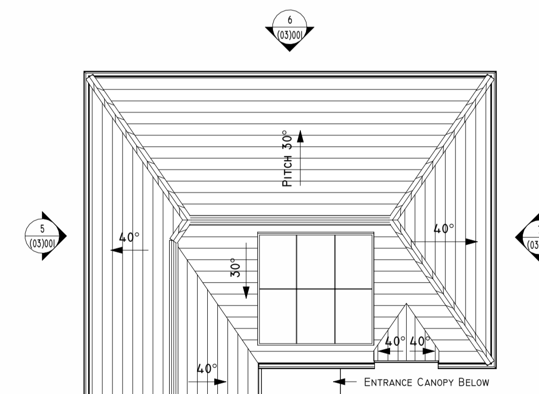
3 ROOF PI 1 : 100
